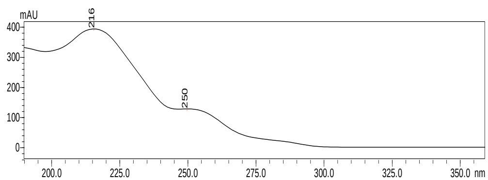
圖十三、五味子素的 UV 圖譜
