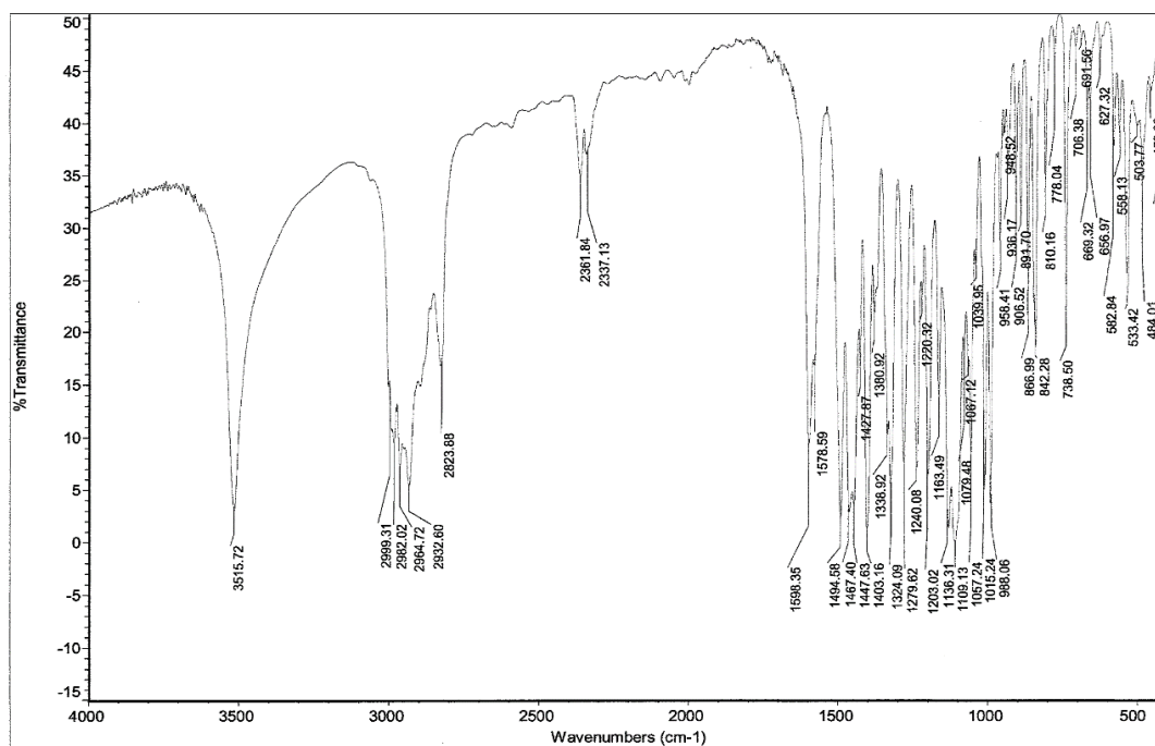
圖十三、五味子素的 FTIR 圖譜
