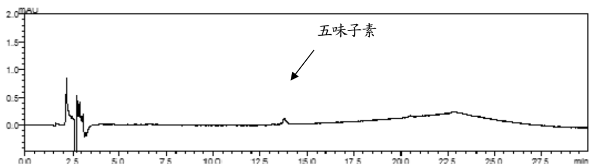
圖四、五味子素之偵測極限層析圖
