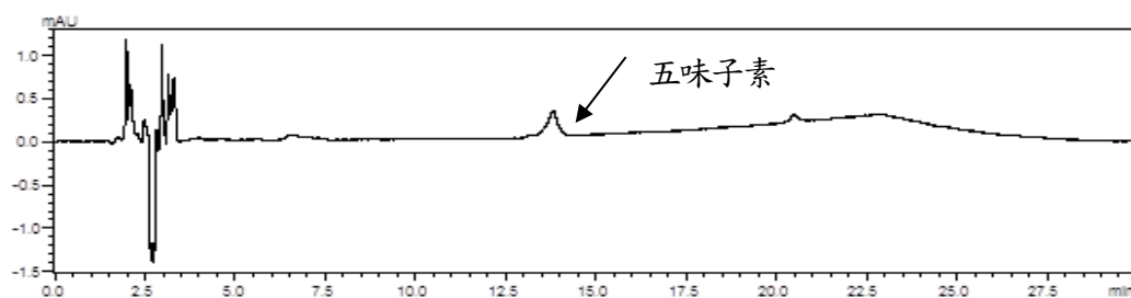
圖五、五味子素之定量極限層析圖
