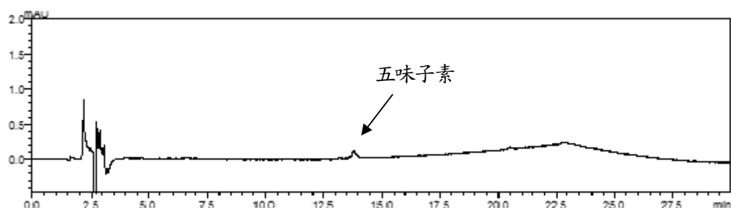
圖四、五味子素之偵測極限層析圖
