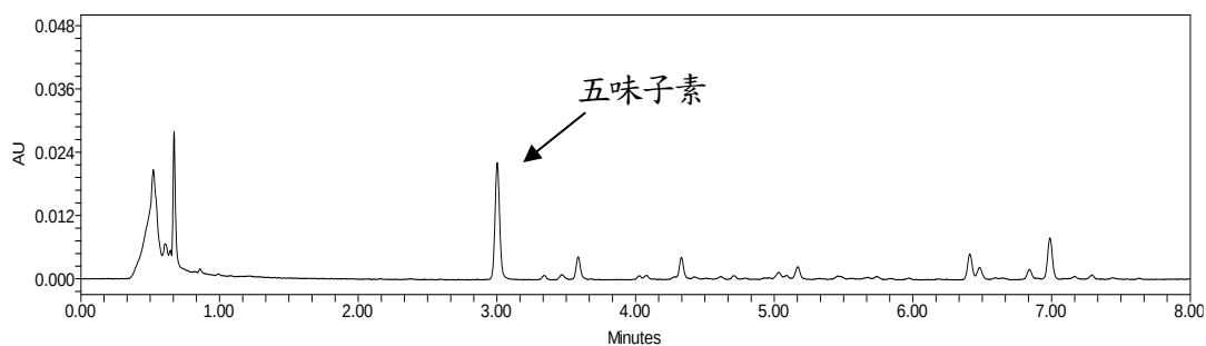
圖八、市售五味子檢品之 UPLC 層析圖
