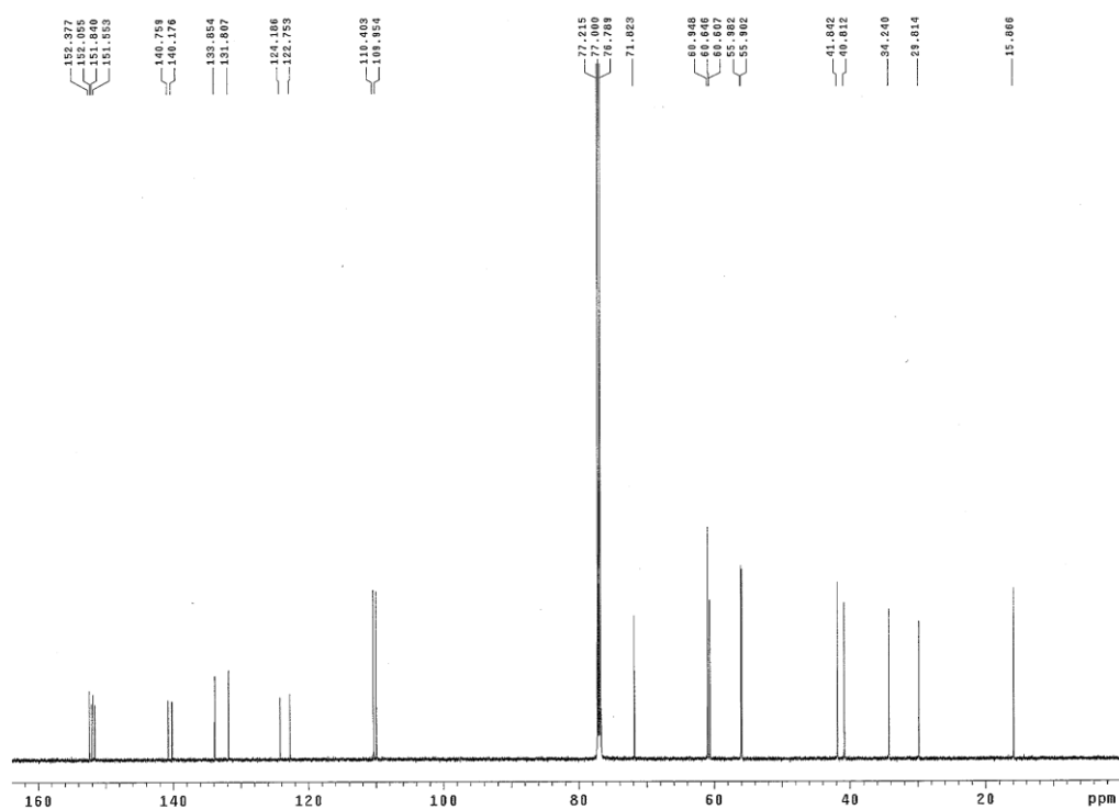
圖十一、五味子素的 ^{13}\text{C} NMR 圖譜( \text{CDCl}_3 )
