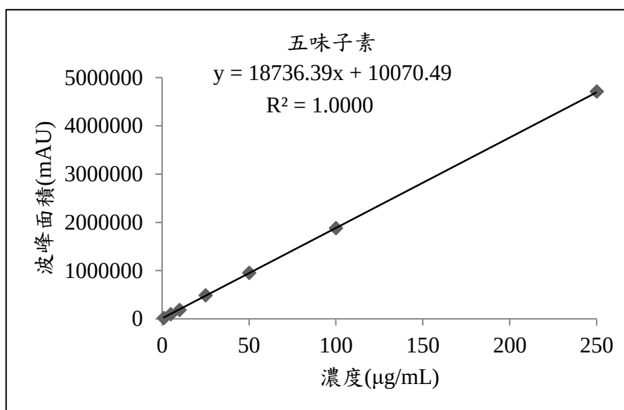
圖三、五味子素之檢量線圖
