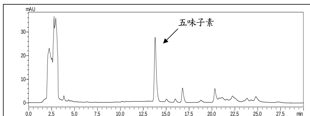
圖二、市售五味子檢品之 HPLC 層析圖
