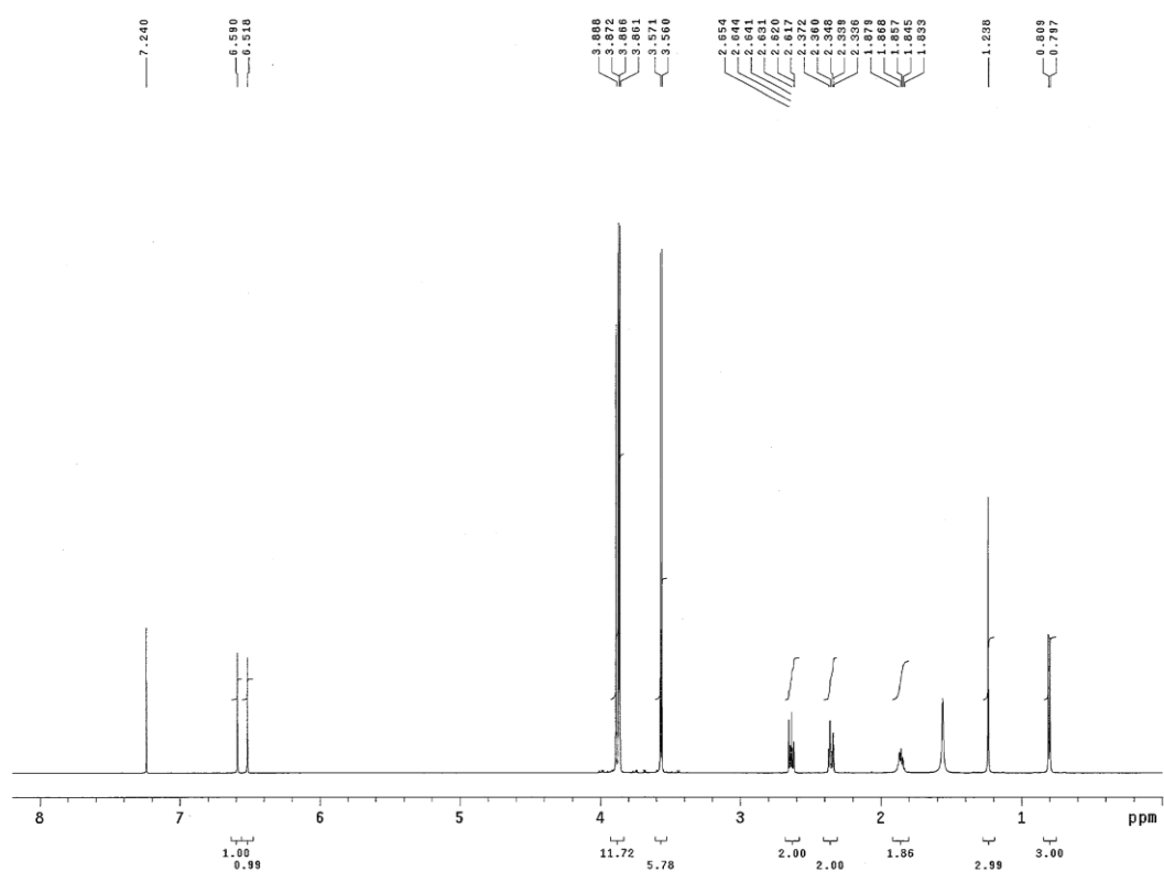
圖十、五味子素的 ^1\text{H} NMR 圖譜( \text{CDCl}_3 )
