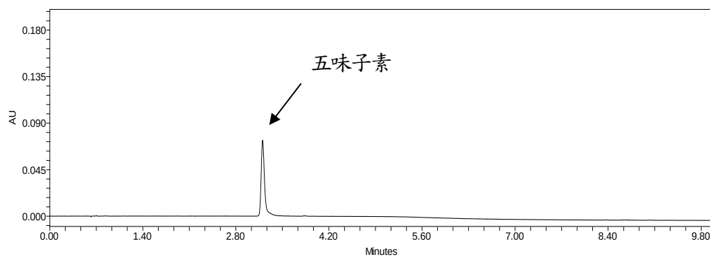
圖六、五味子素標準品溶液之 UPLC 層析圖
