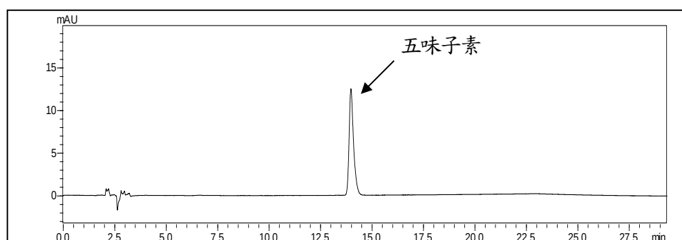
圖一、五味子素標準品溶液之 HPLC 層析圖
