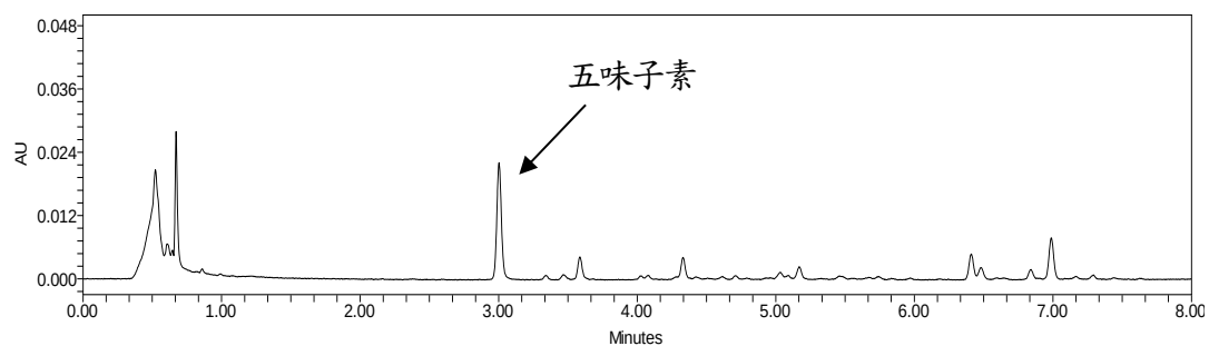
圖七、市售五味子飲片檢品之 UPLC 層析圖
