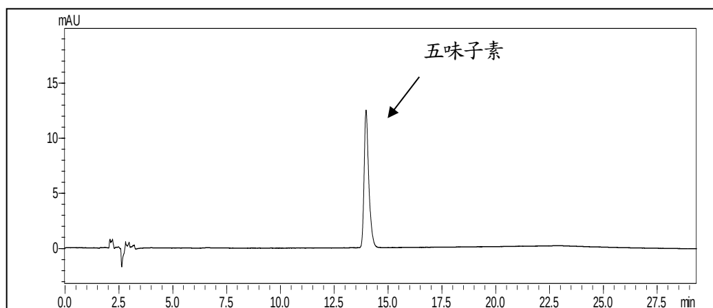
圖一、五味子素標準品溶液之 HPLC 層析圖
