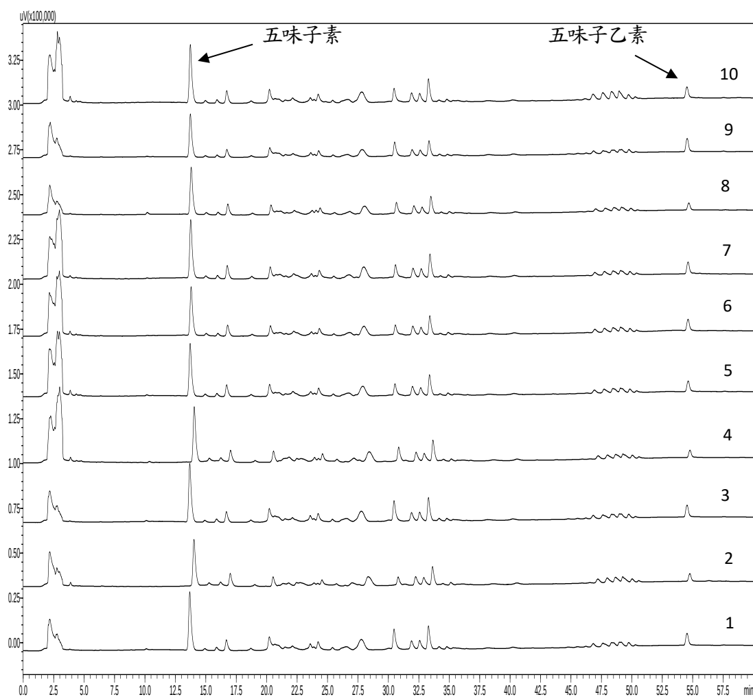
圖六、10 批五味子藥材之 HPLC 指紋圖譜
