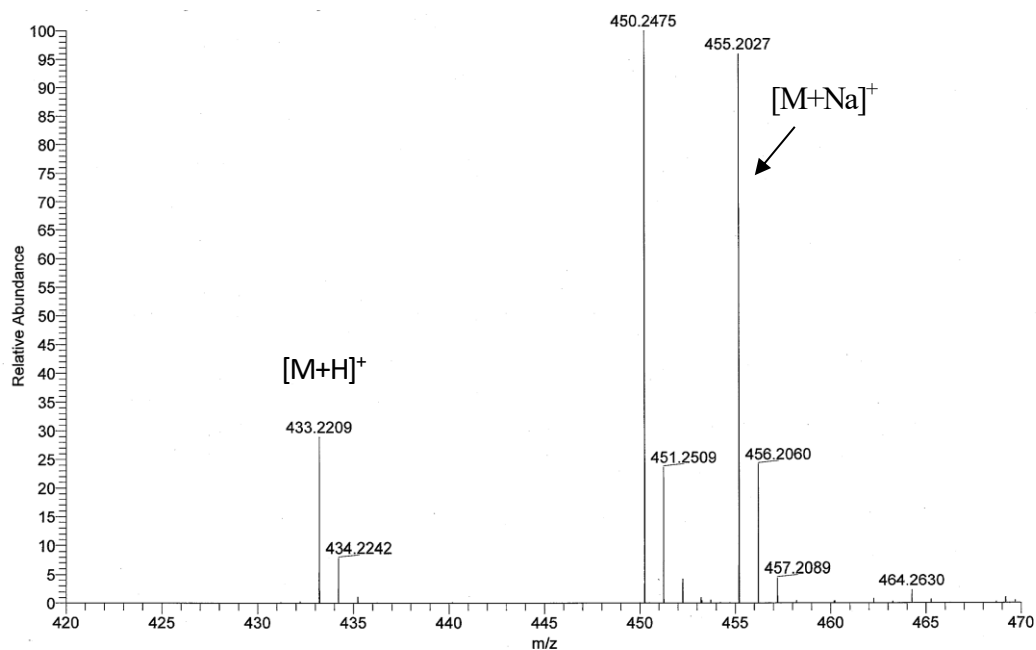
圖十二、五味子素的 ESI-MS 圖譜
