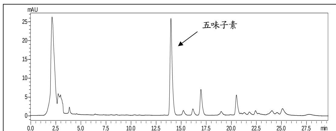
圖二、市售五味子飲片檢品之 HPLC 層析圖
