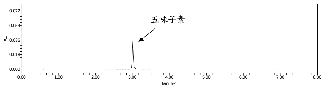
圖七、五味子素標準品溶液之 UPLC 層析圖
